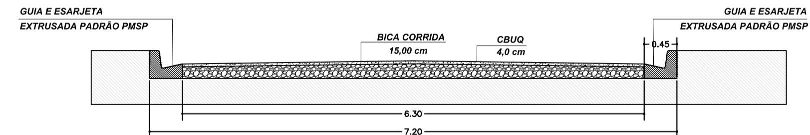
SEÇÃO TRANSVERSAL DA ESTRADA 01 ESCALA 1:50
